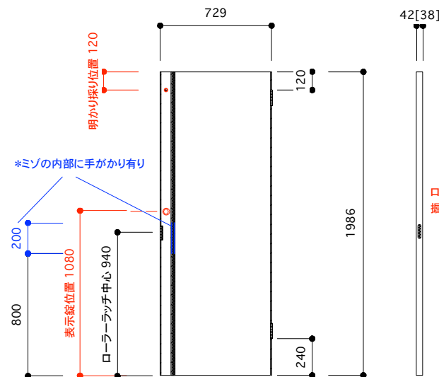
正面図
