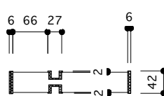
取手・大手 詳細図
