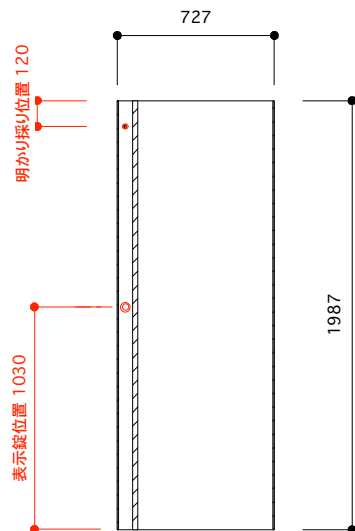
正面図 1/35
