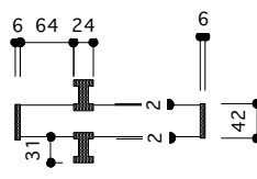
取手・大手 詳細図
