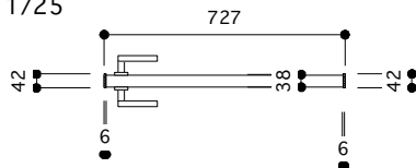
平面図 1/25
