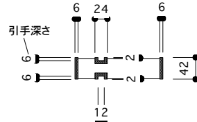
引手・大手 詳細図
