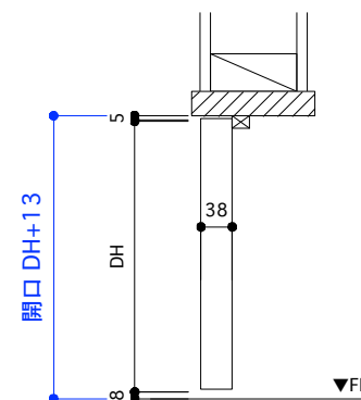
断面図 推奨サイズ
