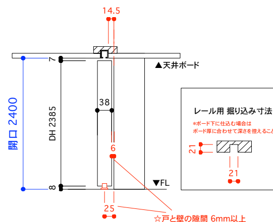
掘り込み有り 埋め込みの場合
