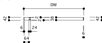
平面図 1/25
