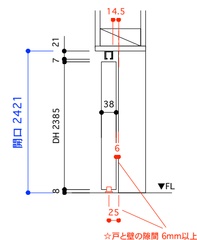
掘り込み無し ベタ付けの場合
