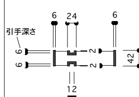
引手・大手 詳細図
