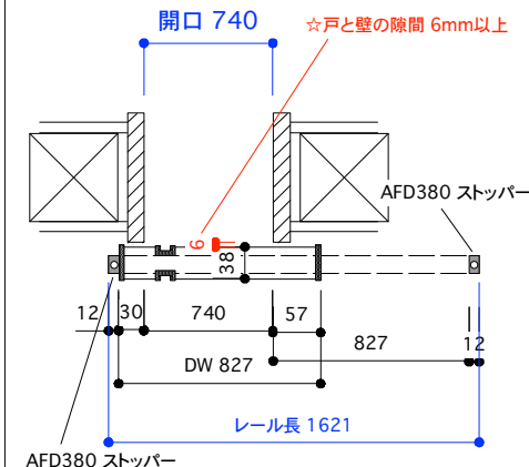
断面図 推奨サイズ
