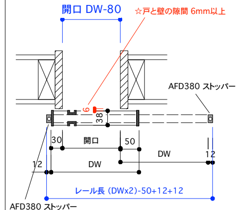
平面図 推奨サイズ[アウトセット仕様]
