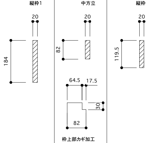
枠詳細図 1/10
