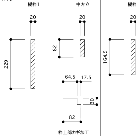
枠詳細図 1/10
