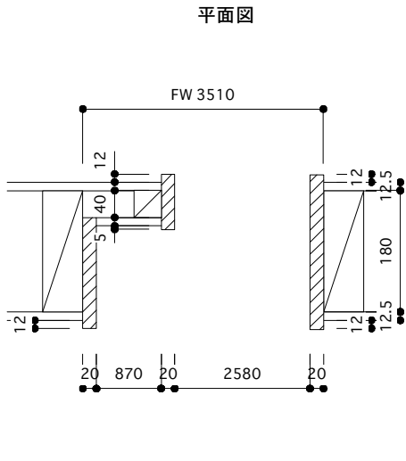
枠詳細図 1/10
